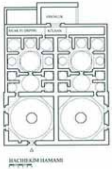
 ek. 19. Hacı Hakim Hamamı planı.
