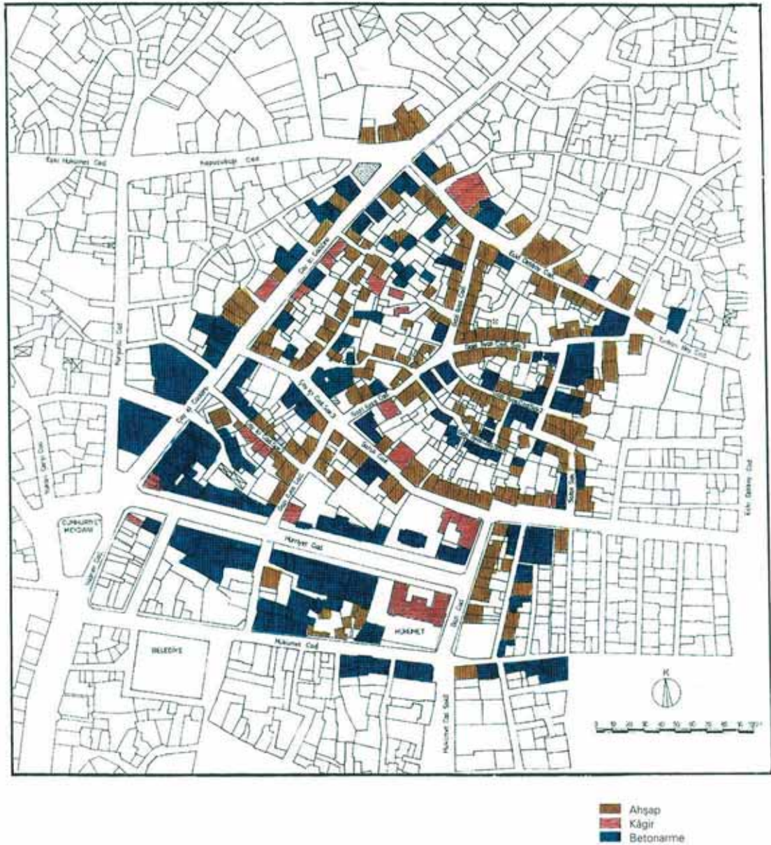
Şek. 7. Edremit ilçe merkezindeki yapıların yapı cinsi analizi.
