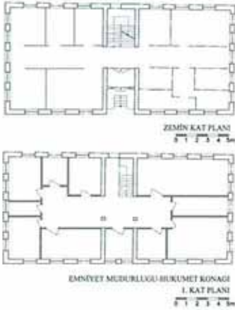
Şek. 14. İlçe Emniyet Müdürlüğü/ eski Hükümet Konağının (env. no: J18.B5.1449) kat planı.
