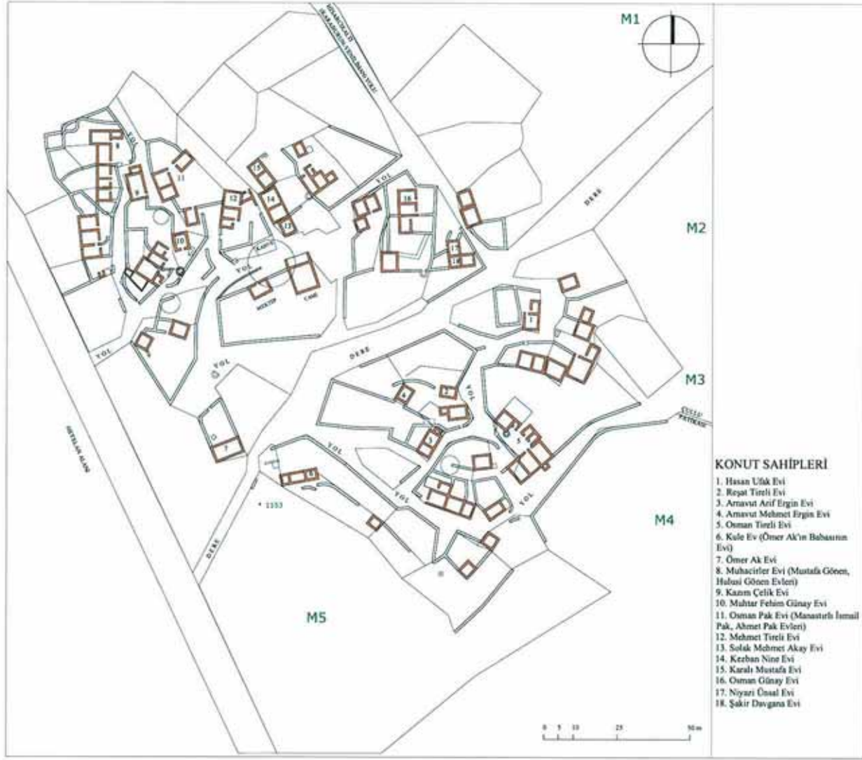
Şek. 1. Hisarcık köyü yerleşim planı (ön restitüsyon, 2004) ve mezarlık alanları (M1, M2, M3, M4).
